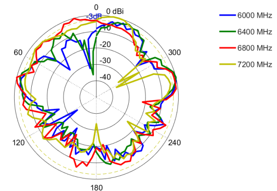
Elevation 2: 6000 – 7200 MHz
